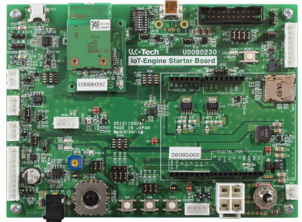
IoT-Engine Starter ボード
