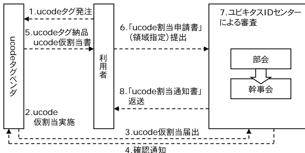
図 21: ucode 仮割当手続きならびに領域指定付 ucode 割当手続きのフロー
