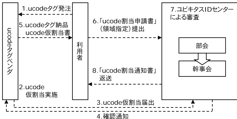
図 20: 領域指定付の ucode 割当申請フロー
