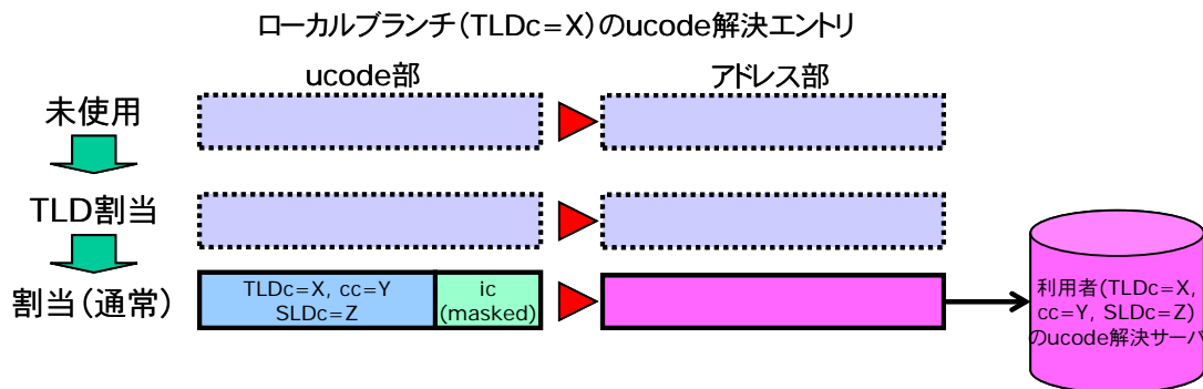
図 13: SLD を管理する ucode 解決エントリの設定 (ローカルブランチが管理)
