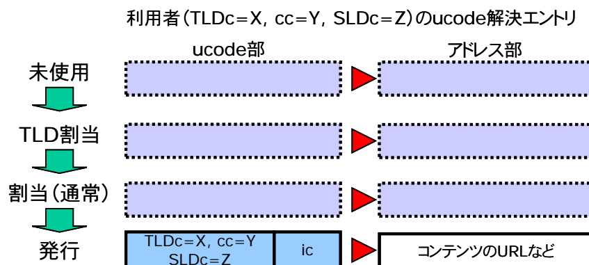
図 14: 識別コード部(ic: identification code)を管理する ucode 解決エントリーの設定 (利用者が管理)
