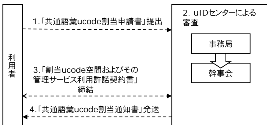
図 12: 共通語彙 ucode 割当申請フロー
