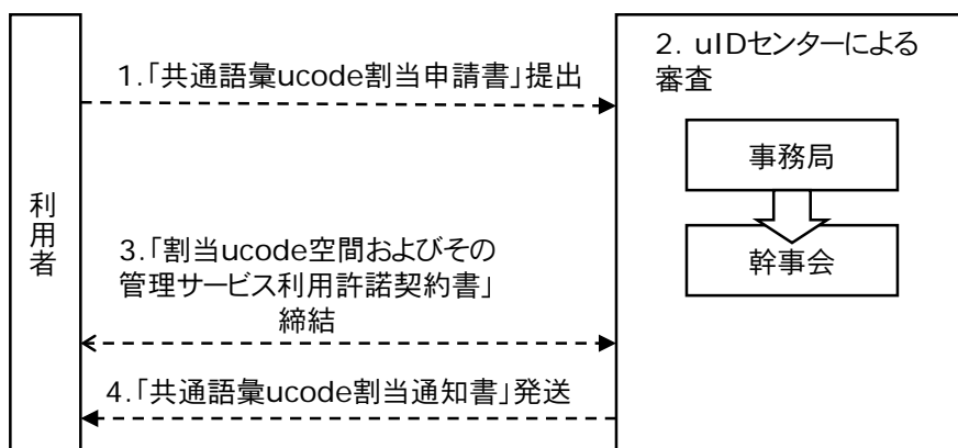
図 22: 共通語彙 ucode 割当申請フロー
