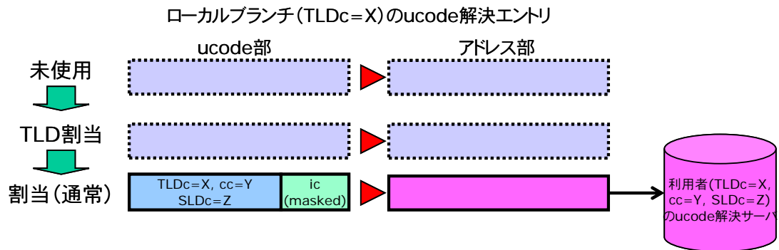
図 19: SLD を管理する ucode 解決エントリーの設定(ローカルブランチが管理)
