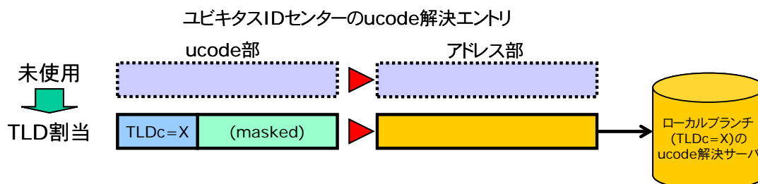
図 17: TLD を管理する ucode 解決エントリの設定 (ユビキタス ID センターが管理)
