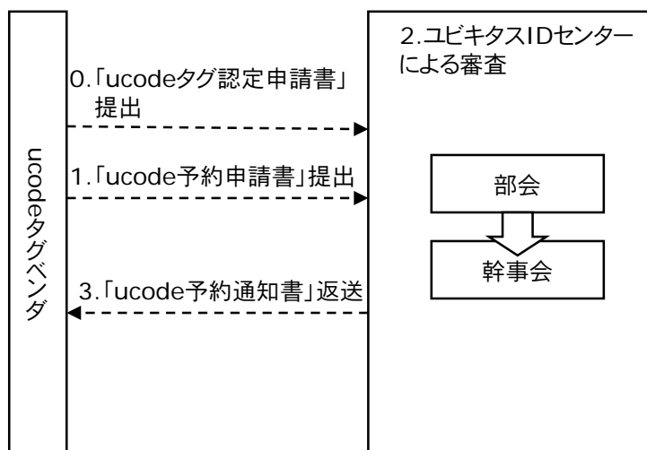
図 15: ucode 予約の手順
